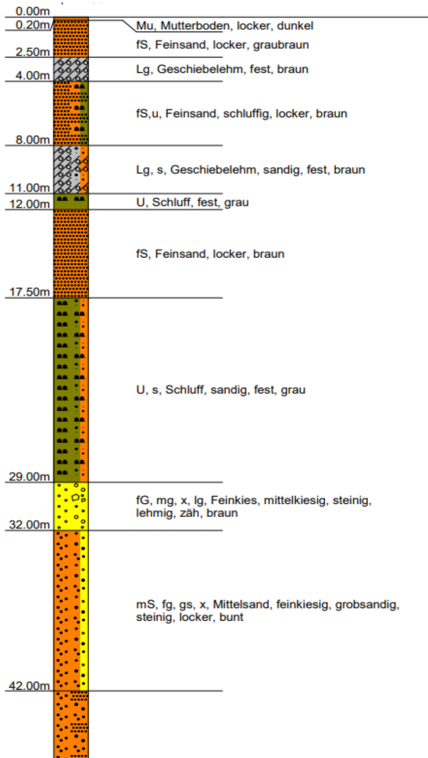
Abb. 1: Vorprofil GWM Biesow 1/26
